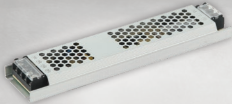
S-300-12V-A LED NAPAJANJE Snaga 300W / 25A Napon 12V Š278*D53*V22mm IP20
