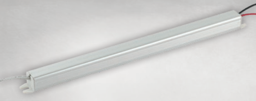
S-48-12V-B LED NAPAJANJE Snaga 48W / 4A Napon 12V Š278*D17*V17mm IP20
