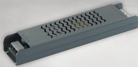
S-300-12V-C LED NAPAJANJE Snaga 300W / 25A Napon 12V Š247*D54*V32mm IP20
