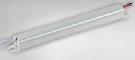
S-24-12V-B LED NAPAJANJE Snaga 24W / 2A Napon 12V Š190*D17*V17mm IP20
