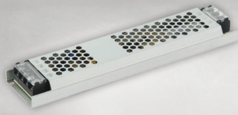
S-100-12V-A LED NAPAJANJE Snaga 100W / 8,5A Napon 12V Š167*D53*V22mm IP20
